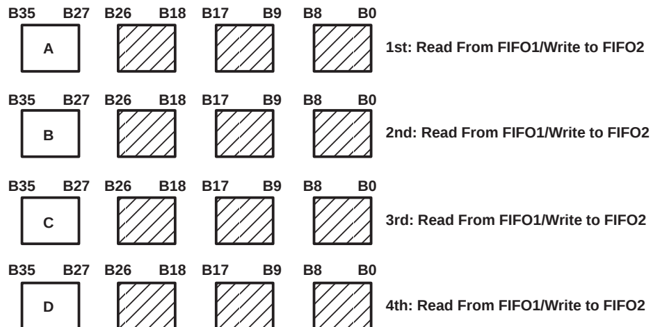
(d) BYTE SIZE – BIG ENDIAN
